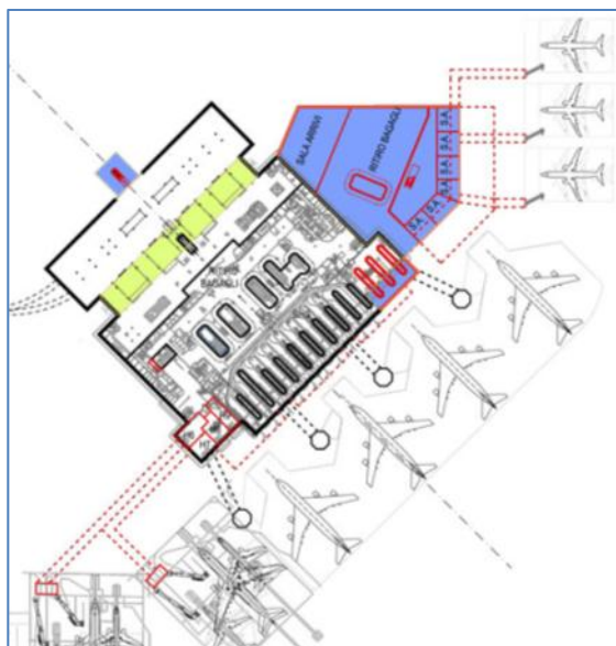
Terminal, livello arrivi, al 2020 I colori evidenziano le aree dove si interviene
