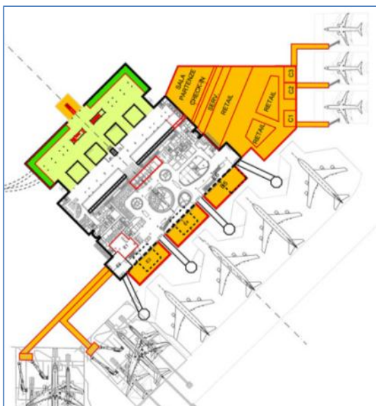
Terminal, livello partenze, al 2020 I colori evidenziano le aree dove si interviene
