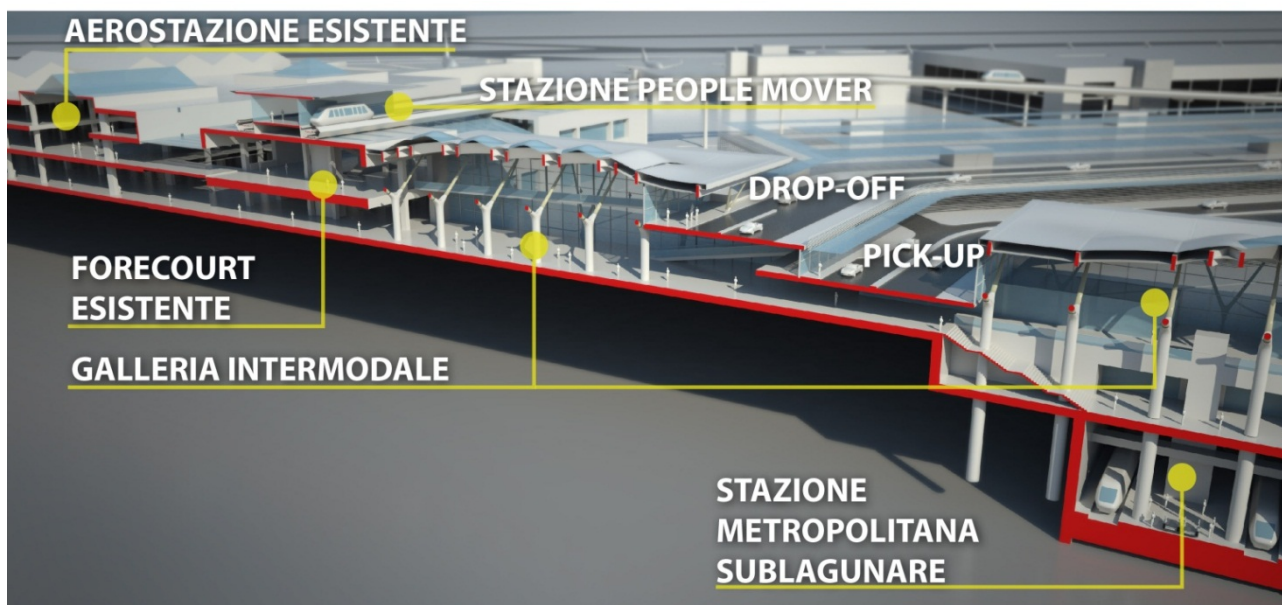
Sezione longitudinale della "Spina" e connessioni intermodali
