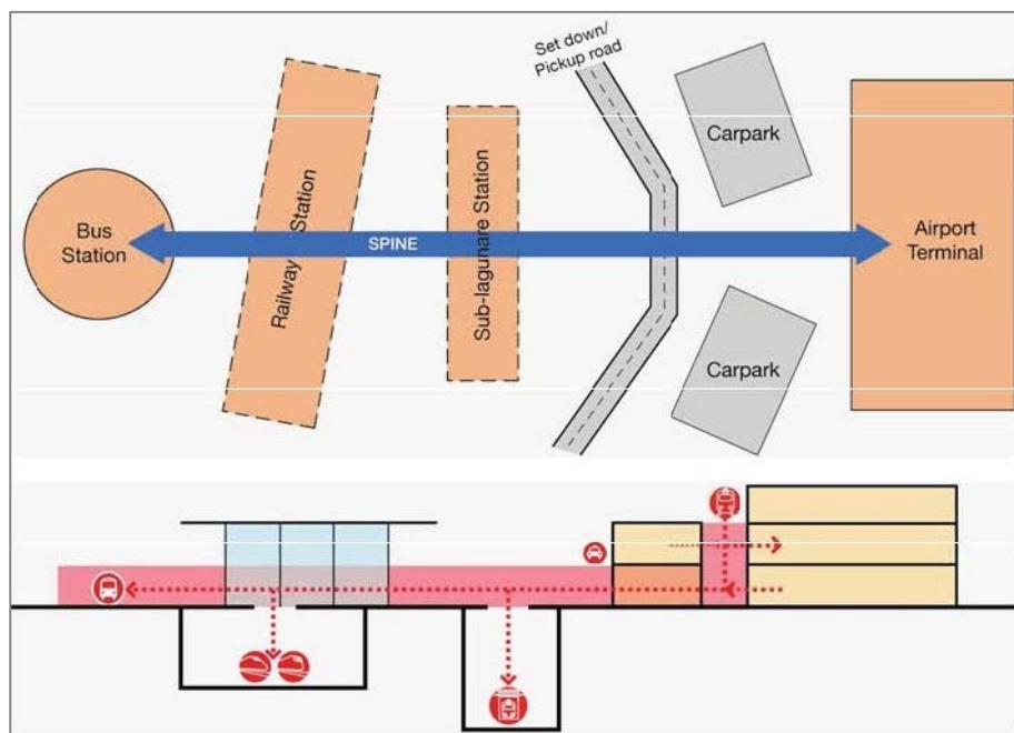
Connessioni intermodali lungo la "Spina"
