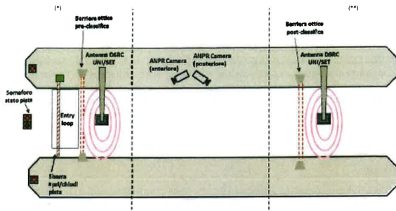
Figura 2 – Schema tipologico della Pista 2.0
