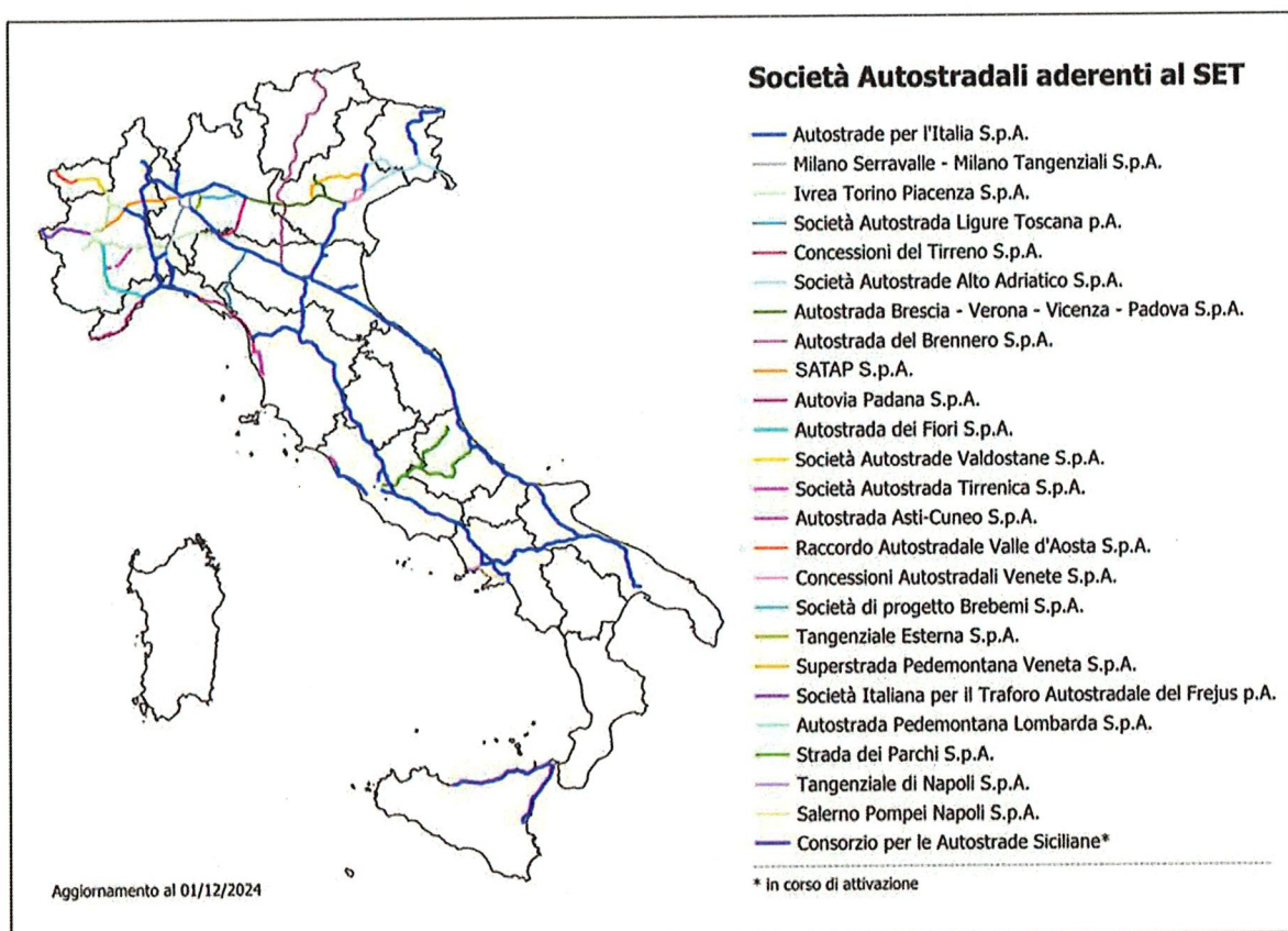
Figura 1: Sviluppo generale della rete autostradale italiana a pedaggio aderente al SET
