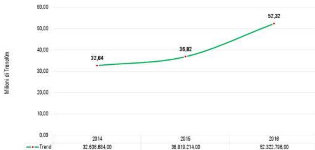
TrenoKm (Ferroviario, Tranvie, Metropolitane, Funicolari) negli anni 2014-2016 - dettaglio regione 'LAZIO'
