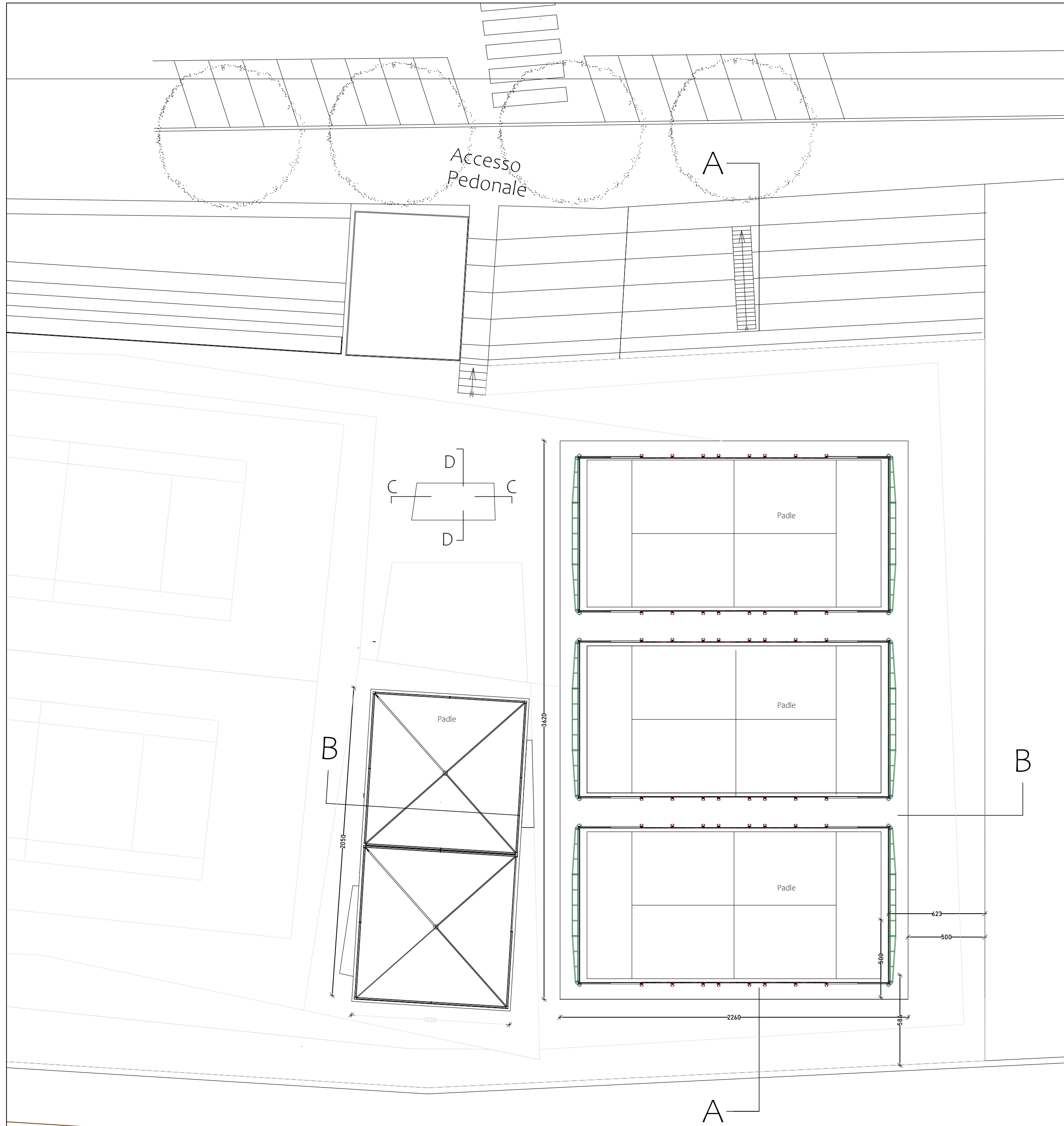
Planimetria Generale 1:100 - Post Operam
