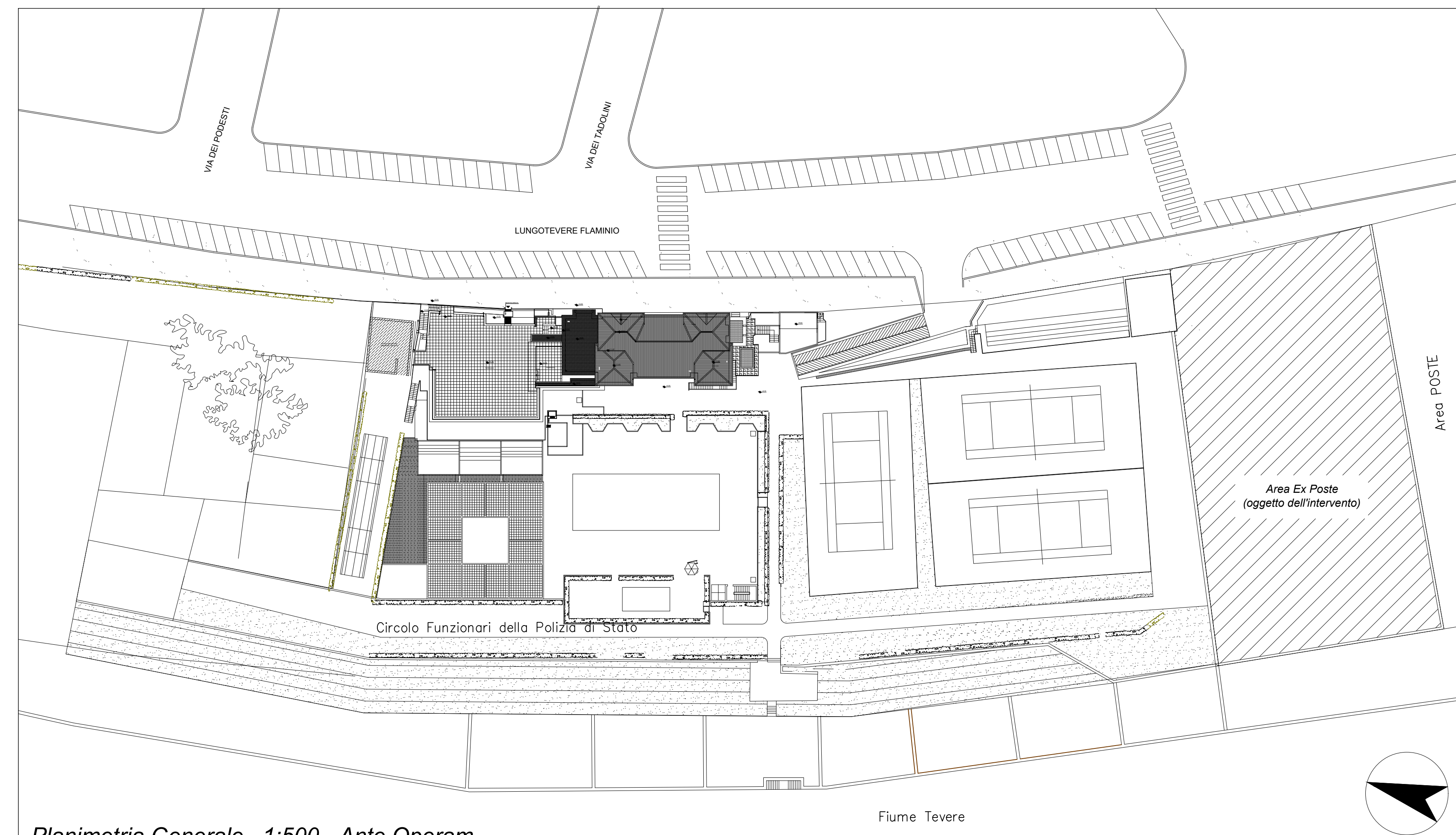
Planimetria Generale 1:500 - Ante Operam
