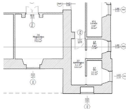
Rilievo geometrico posto a base di gara (coerente con lo stato effettivo dei luoghi)
