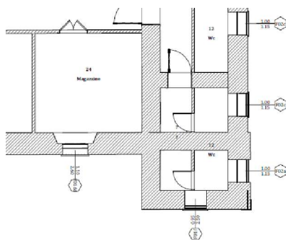
Rilievo geometrico del PFTE
